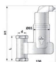
Вертикальное подсоединение
