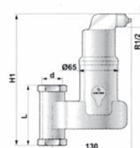
Вертикальное подсоединение
