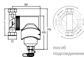
SpiroTrap MB3 доступен с двумя различными присоединениями: 22 мм и 28 мм
