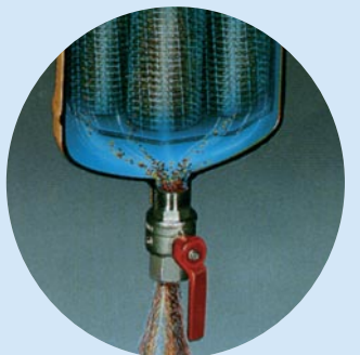
Сброс шлама занимает всего несколько секунд
